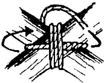
dreifacher Zugbund über den spitzen Winkel
