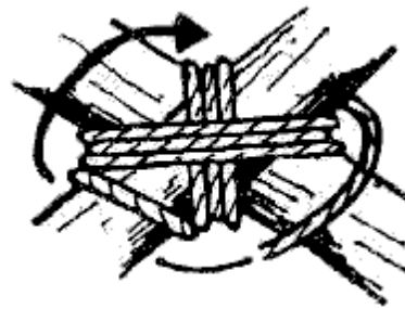
dreifacher Druckbund: Seil rundherum wickeln
