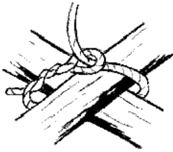
Anfangsknoten: Zimmermannschlag diagonal über beide Stangen
